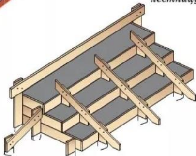
Опалубка под монолитную лестницу
