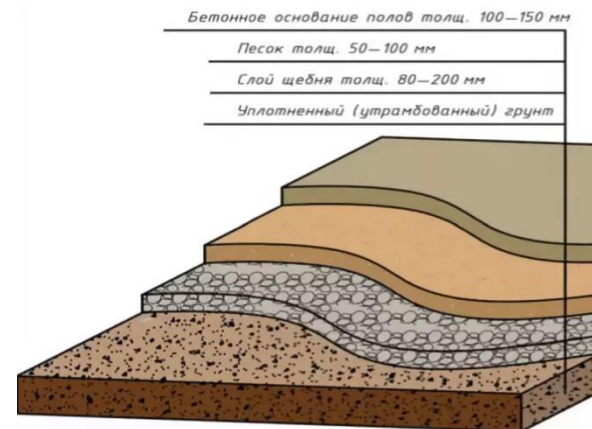
УСТРОЙСТВО БЕТОННОЙ ПЛОЩАДКИ
