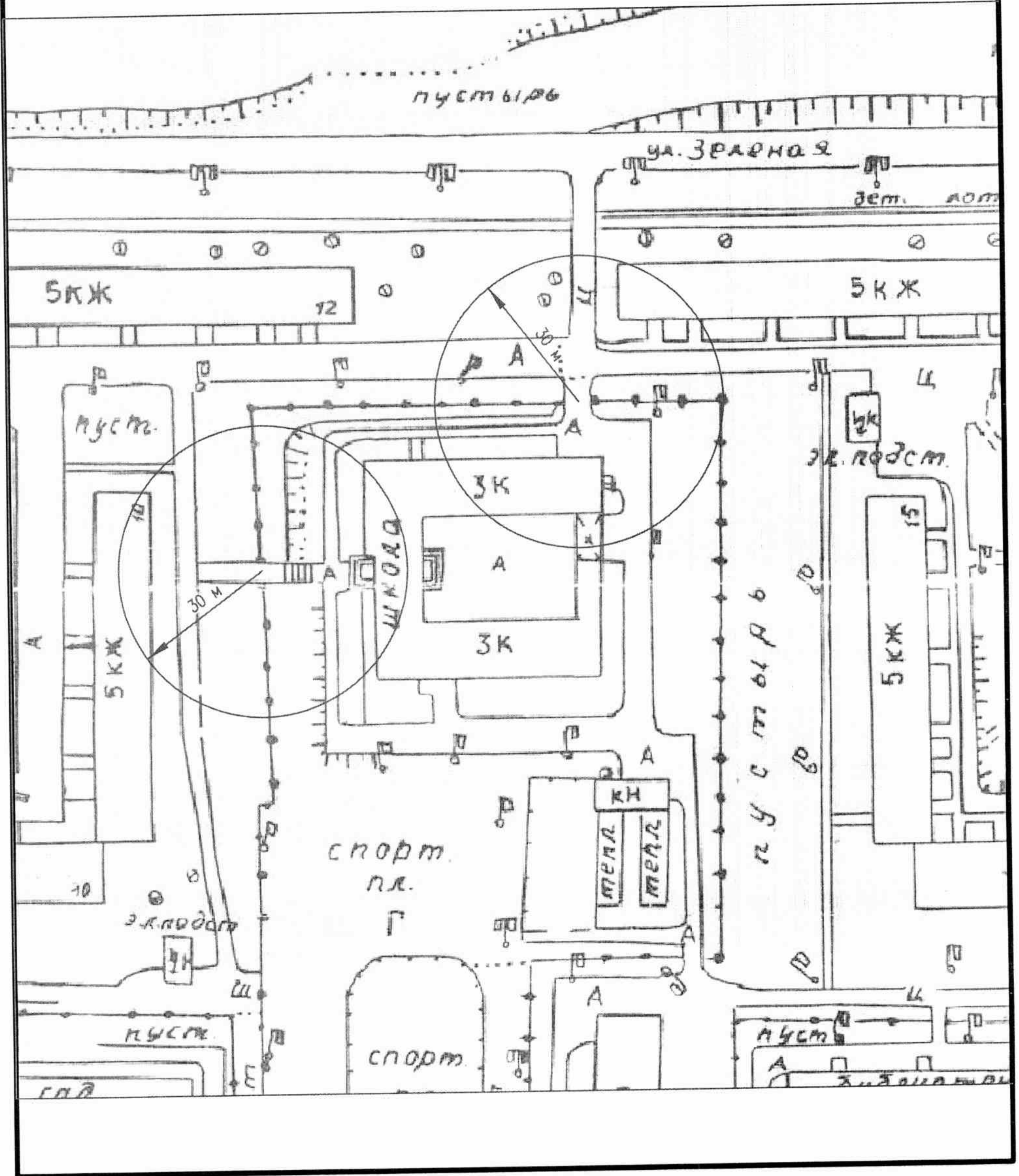
План ситуации в районе здания № 3 в н.п. Коашва М 1:1000
